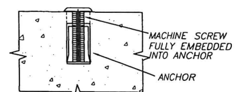
DETAIL A SCALE: 1/2" = 1"
