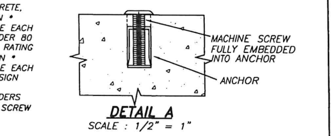
DETAIL A SCALE: 1/2" = 1"
