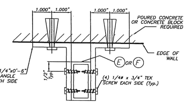
SECTION S1 - S1 SCALE: N. T. S.
